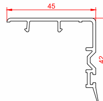
Name: Sliding Door Sash Interlock Code: SWH60-10 Weight: 0.26 kg/m Pkt Qty: 25 pcs
